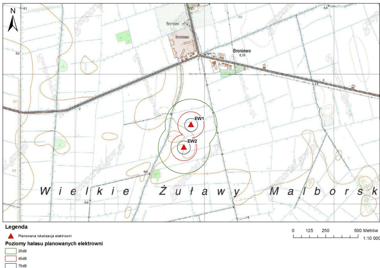
Rysunek 3. Wartości izofon na tle najbliższych zabudowań.
