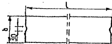
Rys. 1. Wymiarowanie krawężników
