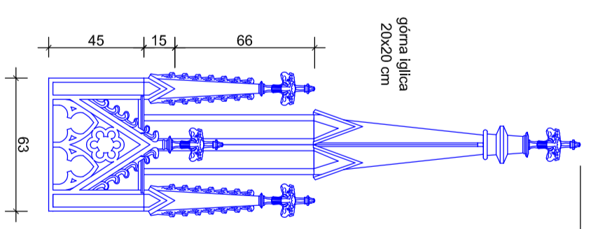
DETAL 1:25
