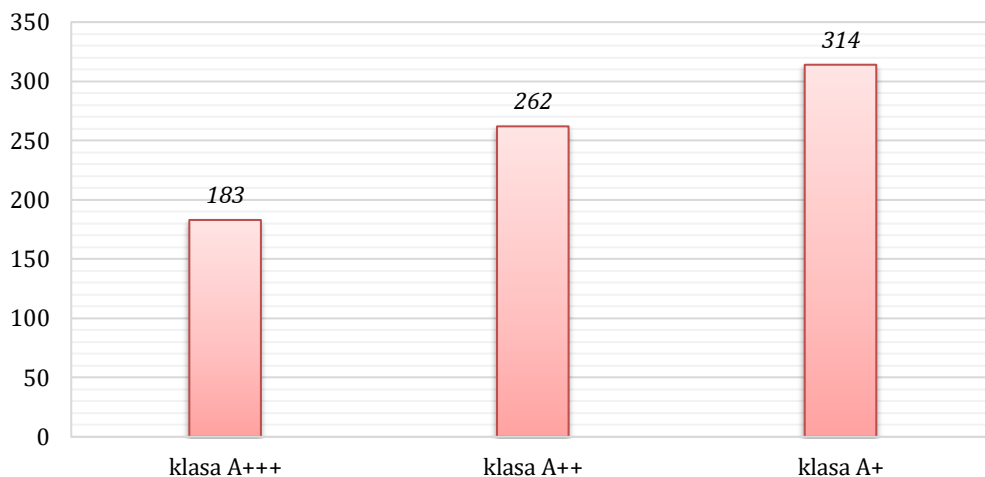
Wykres 45. Porównanie rocznego zużycia energii elektrycznej przez lodówkę w zależności od jej klasy energetycznej [kWh]
