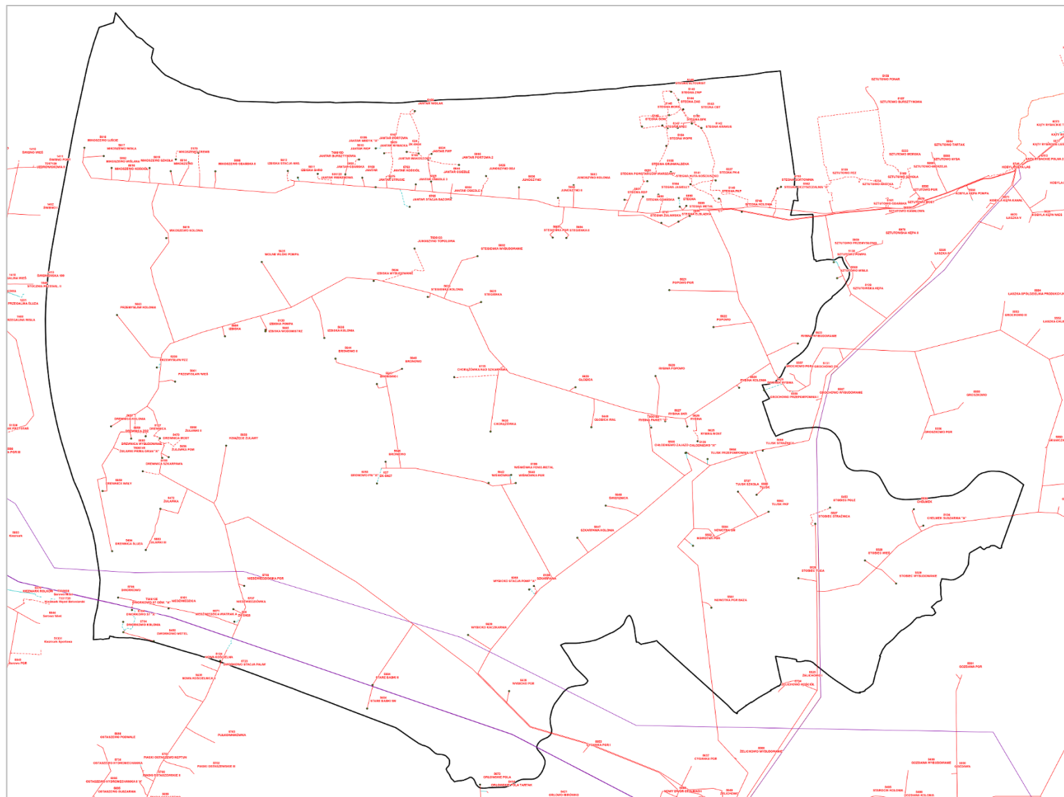
Rysunek 8. Schemat systemu elektroenergetycznego na terenie Gminy Stegna (bez linii niskiego napięcia)
